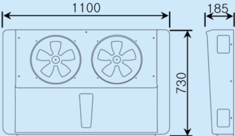
EVAPORADOR
