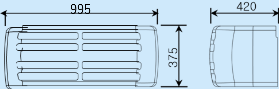
CONDENSADOR
